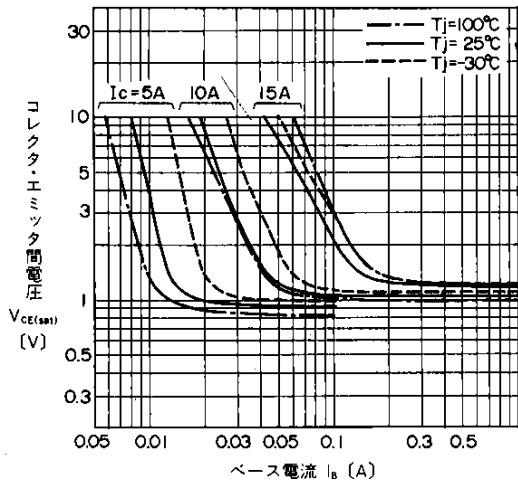
出力特性
