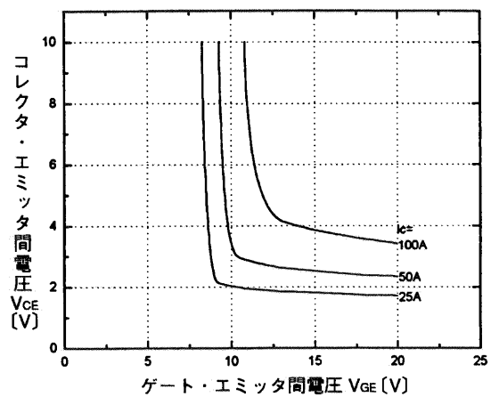
コレクタ・エミッタ間電圧-ゲート・エミッタ間電圧特性 ( T_j=25^{\circ}C ) <ブレーキ部> コレクタ・エミッタ間電圧-ゲート・エミッタ間電圧特性 ( T_j=125^{\circ}C ) <ブレーキ部>
