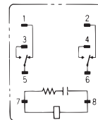
LY2(Z)-CR
