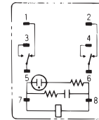
LY2(Z)N-CR
