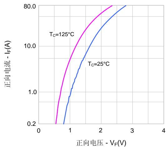
图12. 正向特性
